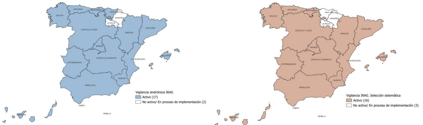
Figura 2. Implementación de la vigilancia de IRAG en España. Componente sindrómico (izquierda) y de selección sistemática (derecha). SiVIRA, temporada 2023-2024.
