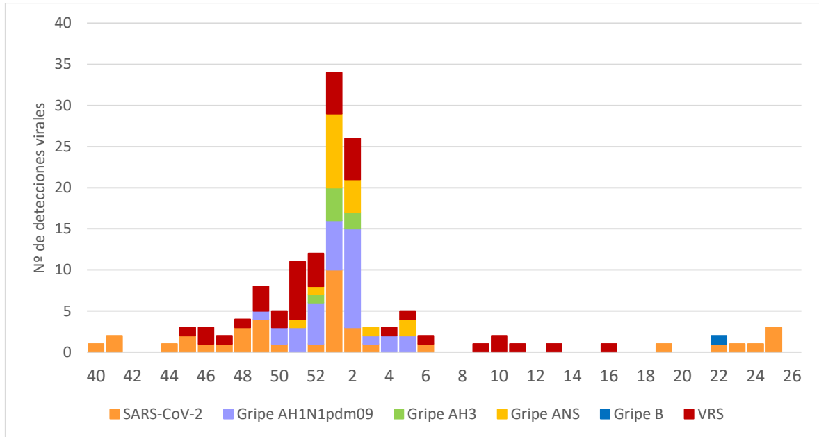
Figura 22. Número de detecciones de SARS-CoV-2, gripe y VRS. Sistema de vigilancia de IRAG del área I de salud, componente sistemático. Temporada 2023/2024. Región de Murcia.
