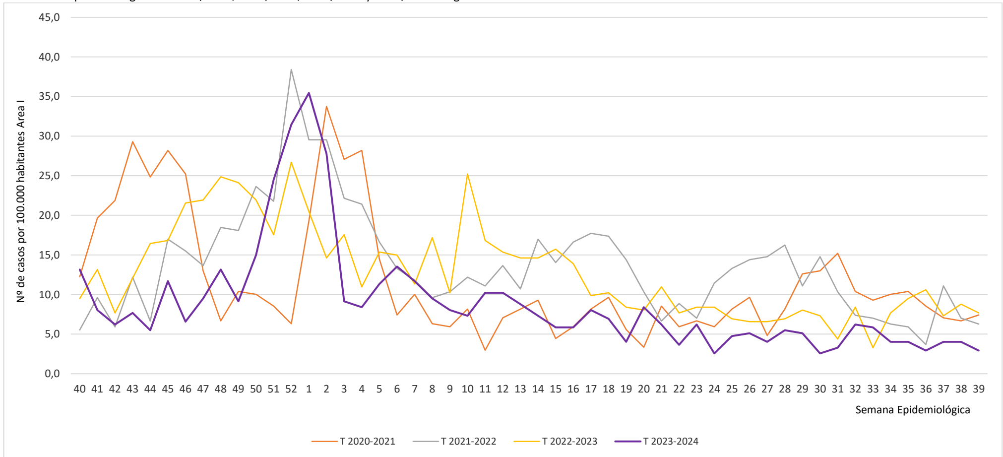
Figura 18. Evolución de la incidencia acumulada de IRAG según temporada de vigilancia. Sistema centinela de Vigilancia de las IRAG, componente sindrómico. Temporadas vigiladas: 2020/2021; 2021/2022; 2022/2023 y 2023/2024. Región de Murcia.
