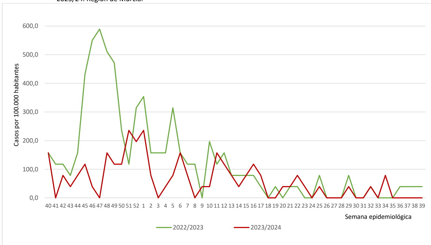
Figura 21. Evolución de la incidencia acumulada semanal de IRAG entre los menores de 1 año. Vigilancia centinela de casos hospitalizados de IRAG del Área I de Salud, componente sindrómico. Temporada 2023/24. Región de Murcia.
