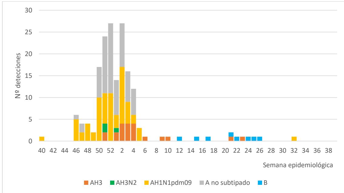
Figura 16. Subtipos de gripe identificados semanalmente. Sistema de vigilancia de IRA en Atención Primaria, red centinela sanitaria de la Región de Murcia. Temporada 2023/24.
