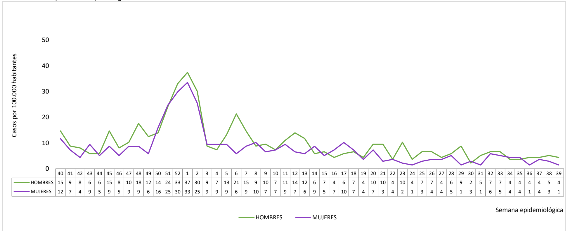
Figura 19. Evolución de la incidencia acumulada semanal de IRAG según sexo. Vigilancia centinela de casos hospitalizados de IRAG del Área I de Salud, componente sindrómico. Temporada 2023/24. Región de Murcia.
